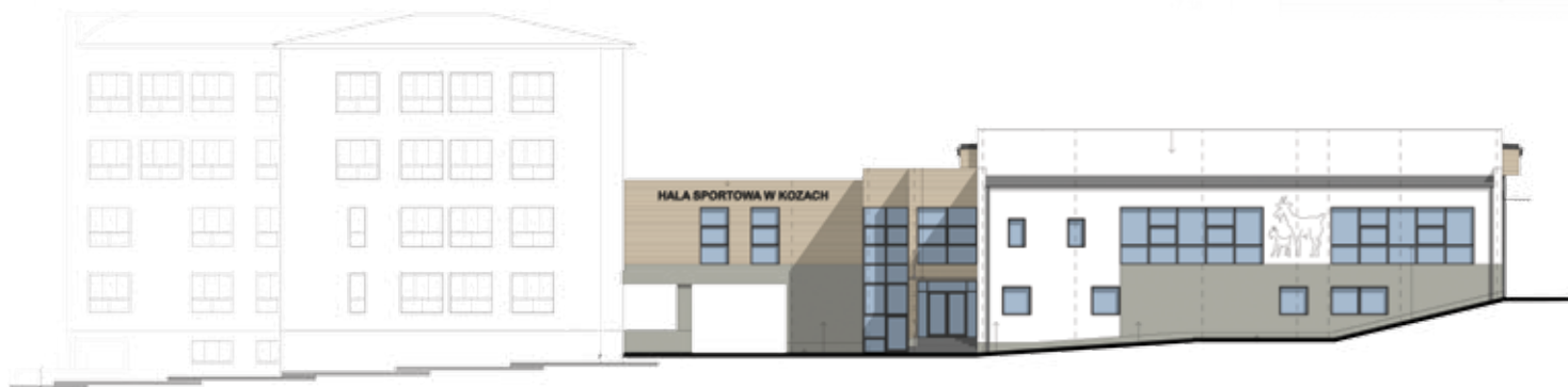
Elewacja od strony zachodniej (widok od boiska do koszykówki)
